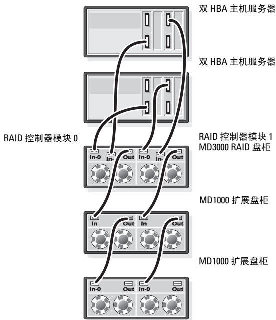
图 3-2. 直接连接的 SAS 群集中的布线
