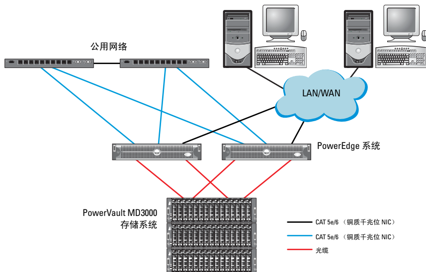
图 3-1. 串行连接 SCSI (SAS) 群集和 Dell PowerVault MD3000 的布线
