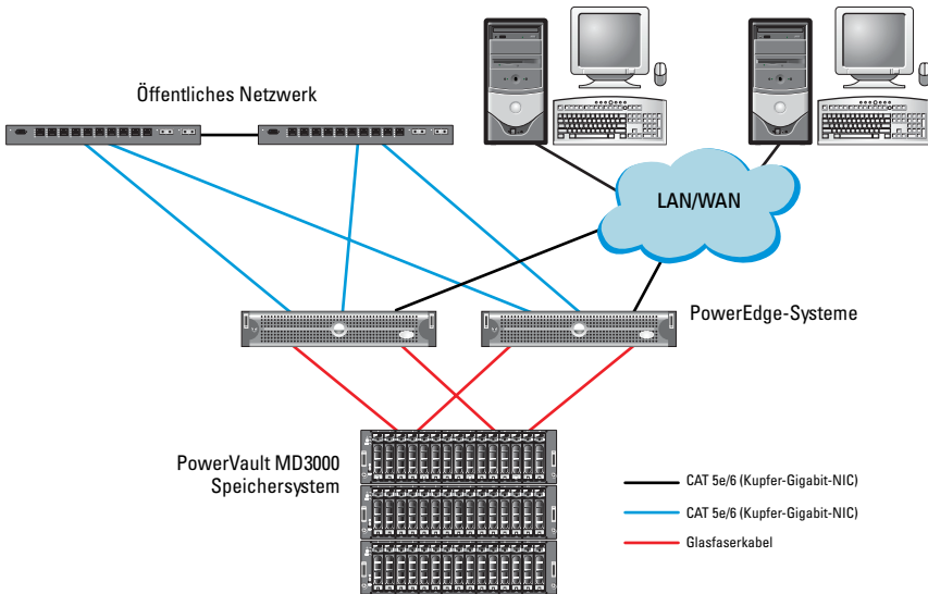
Abbildung 3-1. Verkabelung des SAS (Serial-Attached SCSI)-Clusters und des Dell PowerVault MD3000
