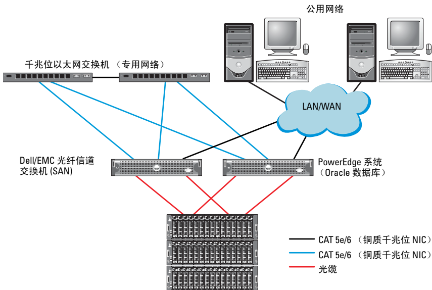
图 2-1. SAN 连接的光纤信道群集的硬件连接。
