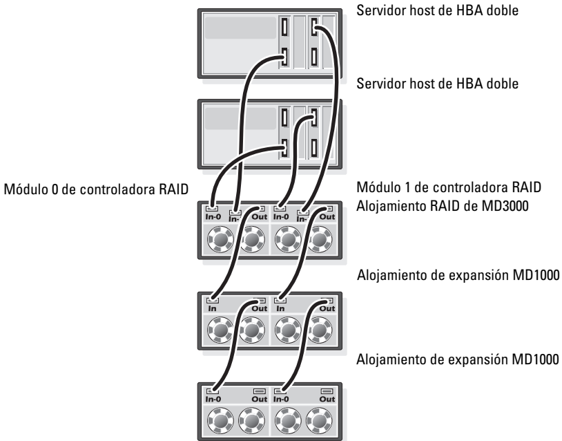
Ilustración 3-2. Cableado de un clúster SAS de conexión directa
