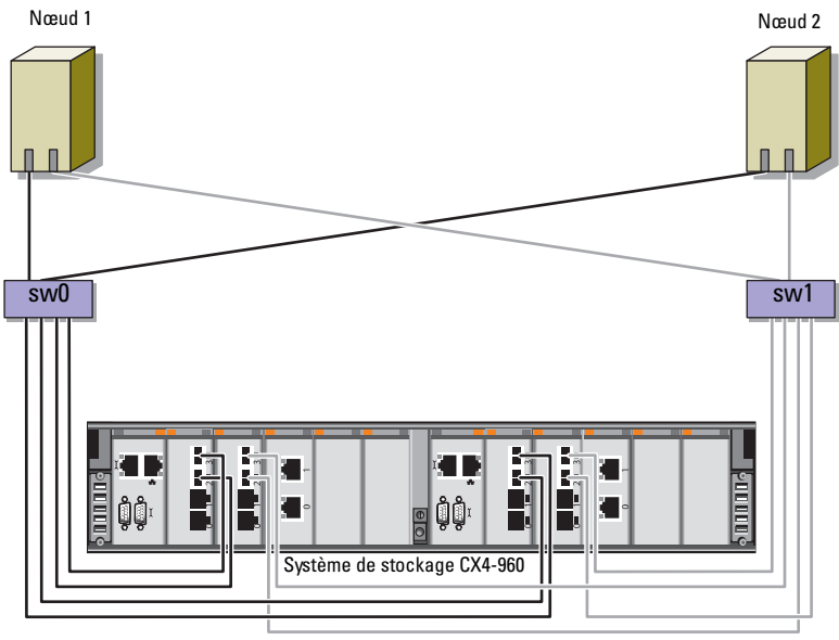
Figure 2-2. Câblage d'un cluster Fibre Channel Dell/EMC connecté à un SAN
