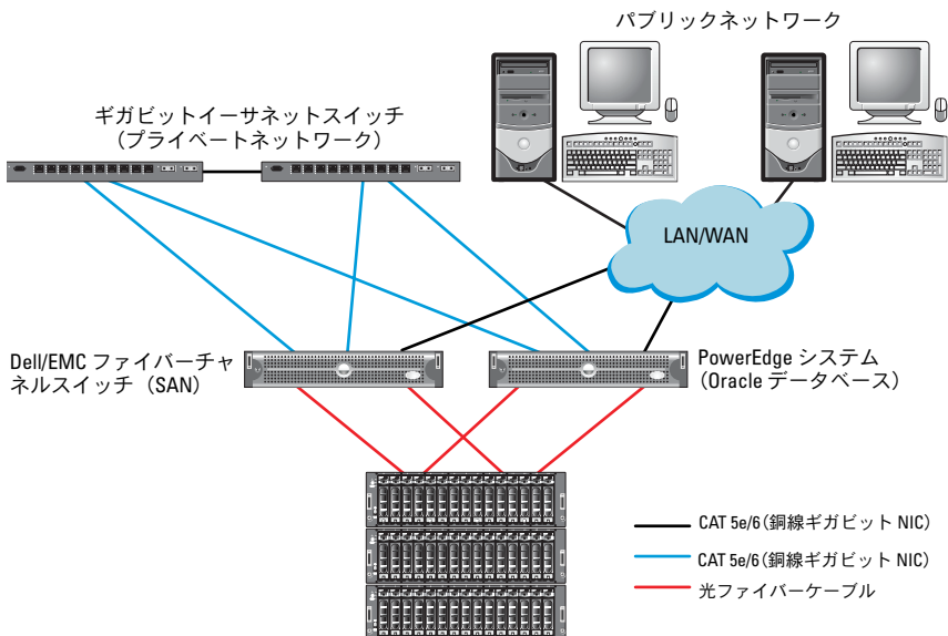
図 2-1. SAN 接続のファイバーチャネルクラスタ用のハードウェア接続
