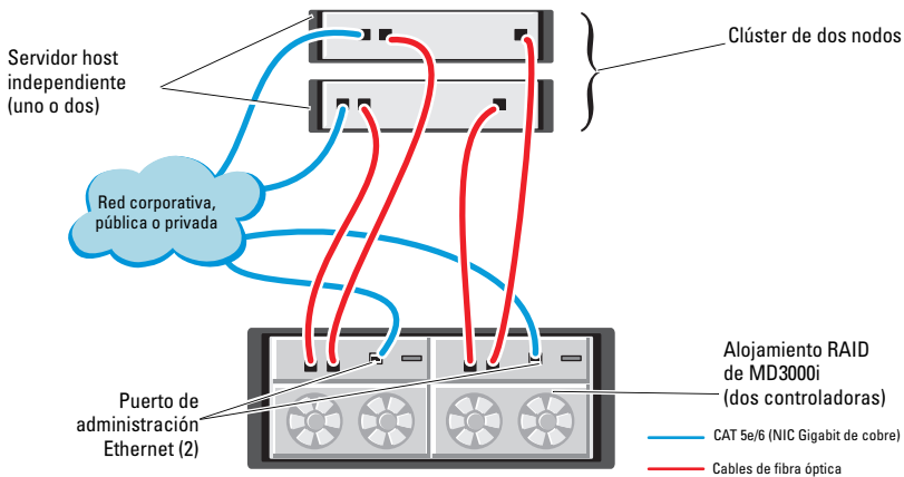
Ilustración 4-1. Cableado de los clústeres iSCSI de conexión directa
