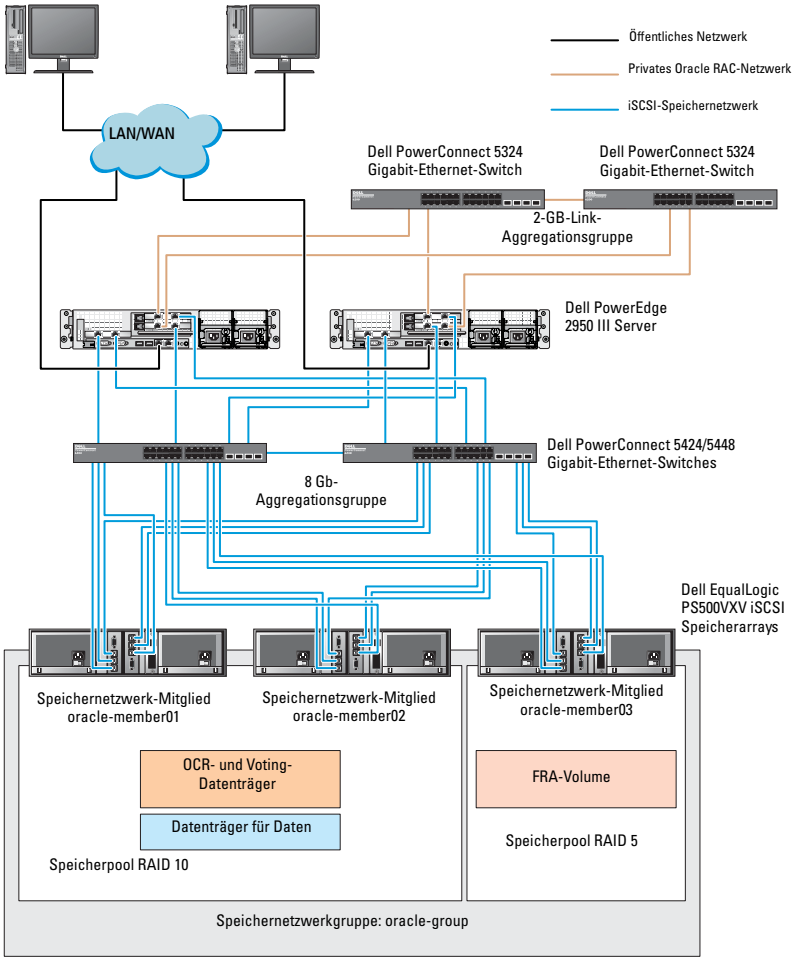
Abbildung 5-2. Oracle RAC-Beispielkonfiguration mit drei PS5000XV-Arrays
