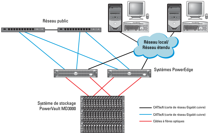
Figure 3-1. Câblage du cluster SAS et du système Dell PowerVault MD3000
