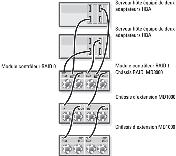
Figure 3-2. Câblage d'un cluster SAS à connexion directe
