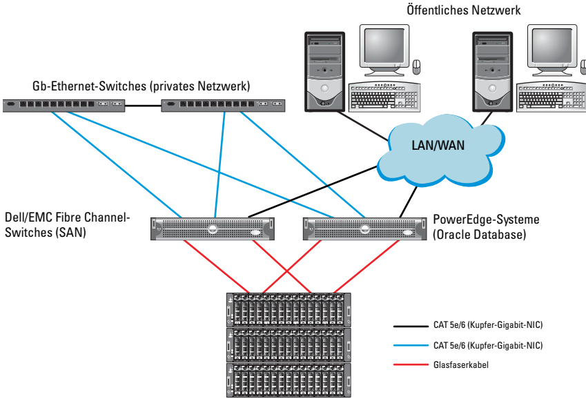
Abbildung 2-1. Hardwareverbindungen für einen SAN-Attached Fibre-Channel-Cluster
