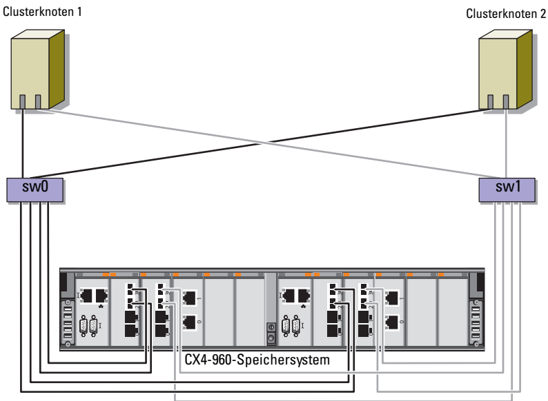
Abbildung 2-2. Verkabeln eines Dell/EMC SAN-Attach-Fibre-Channel-Clusters
