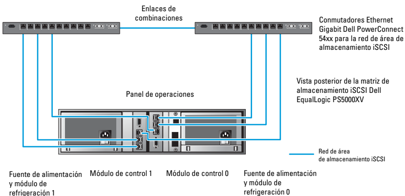
Ilustración 5-1. Configuración de red recomendada
