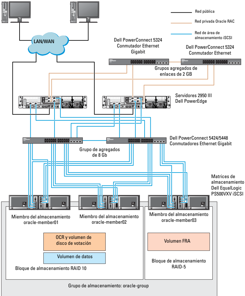
Ilustración 5-2. Configuración de Oracle RAC de muestra con tres matrices PS5000XV
