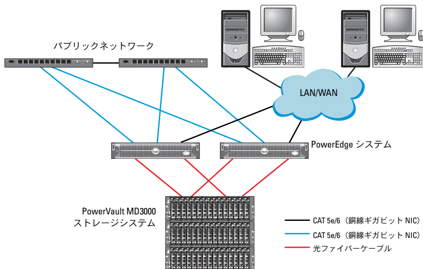
図 3-1. SAS (シリアル接続 SCSI) クラスタと Dell PowerVault MD3000 のケーブル接続
