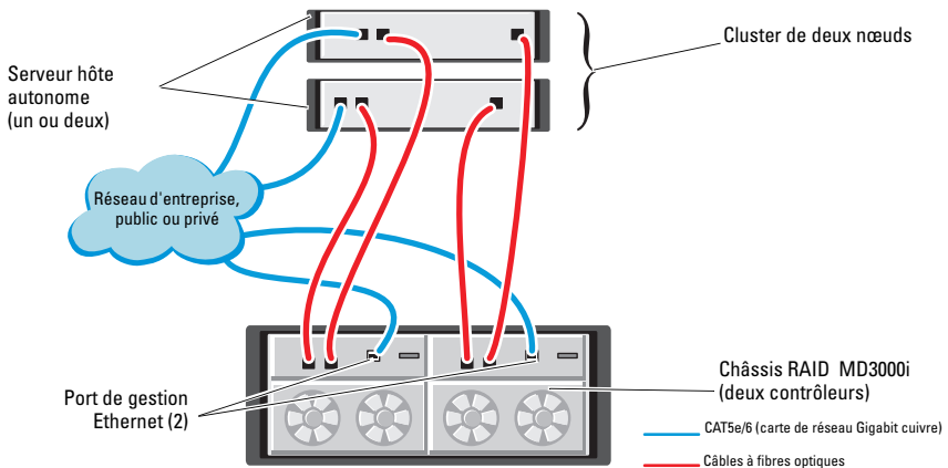
Figure 4-1. Câblage de clusters iSCSI à connexion directe
