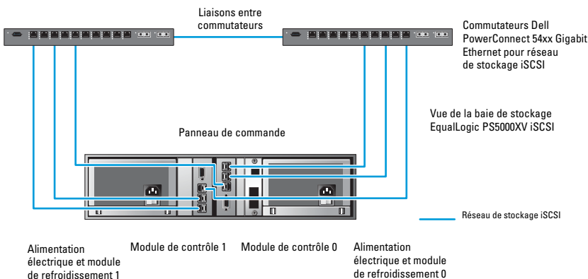
Figure 5-1. Configuration réseau recommandée
