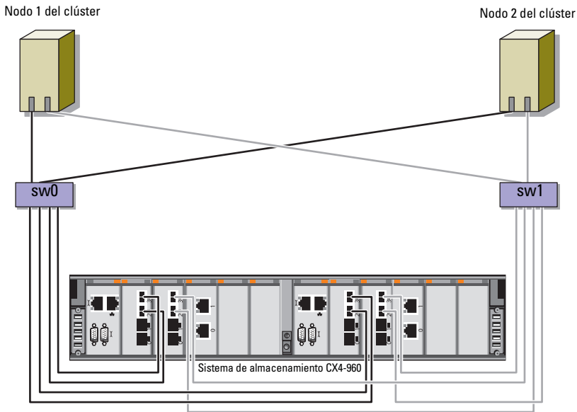
Ilustración 2-2. Cableado de un clúster Dell/EMC Fibre Channel de conexión mediante SAN
