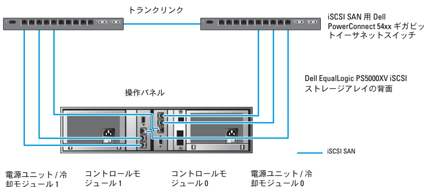
図 5-1. 推奨ネットワーク構成
