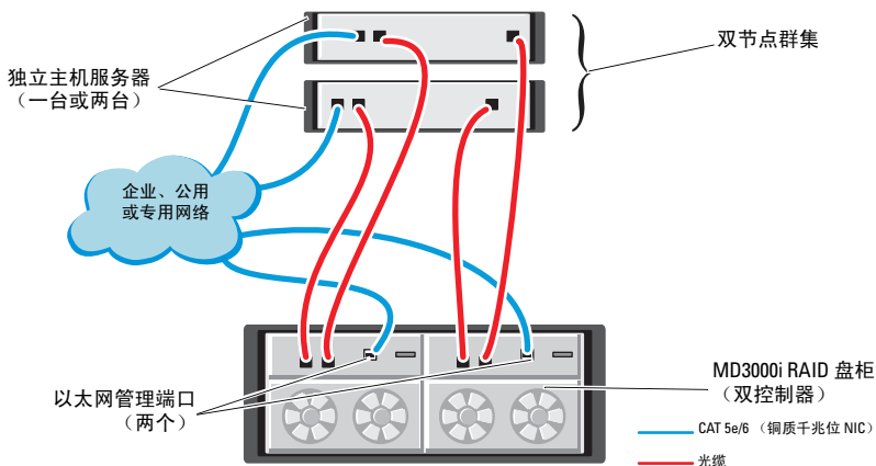
图 4-1. iSCSI 直接连接群集布线
