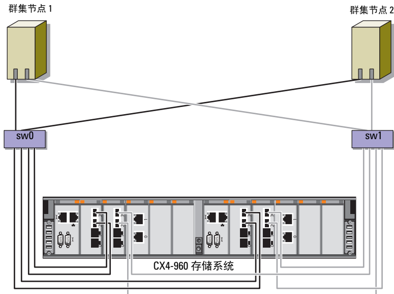
图 2-2. 在 Dell/EMC SAN 连接光纤信道群集中布线
