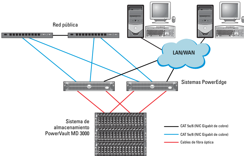
Ilustración 3-1. Cableado del clúster SCSI (SAS) de conexión serie y Dell PowerVault MD3000
