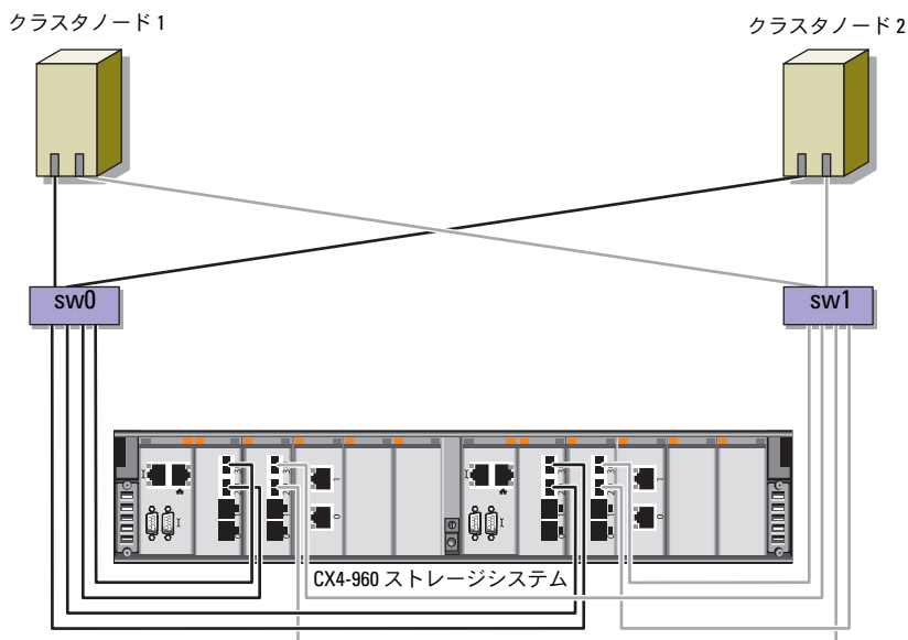
図 2-2. SAN 接続の Dell/EMC ファイバーチャネルクラスタのケーブル接続
