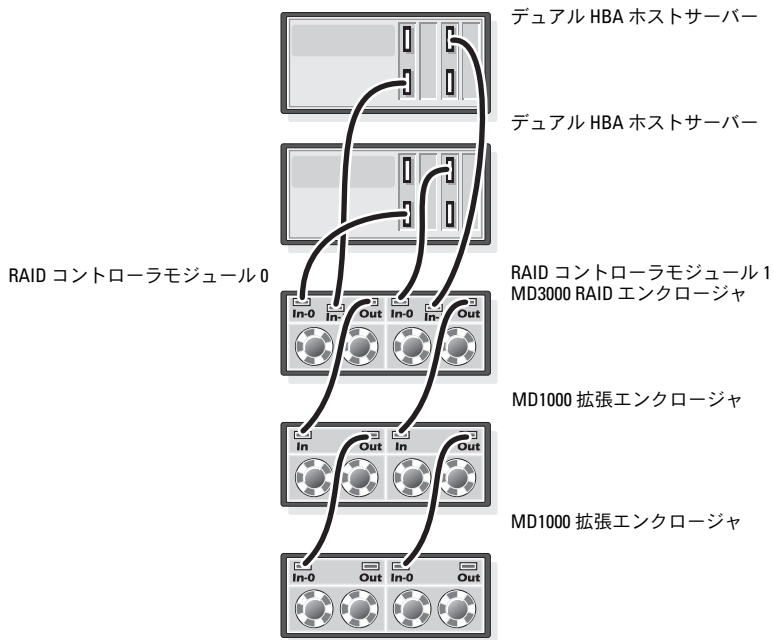
図 3-2. 直接接続 SAS クラスターのケーブル接続
